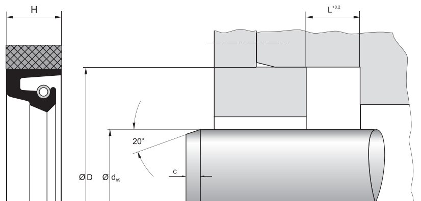
沟槽尺寸系列表MF1
